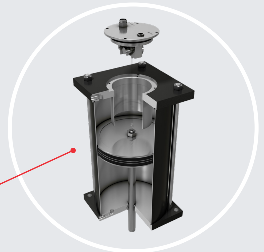
Modèle AT de Cowan
